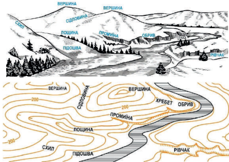
Іл. 33.2. Зображення рельєфу місцевості горизонталями
