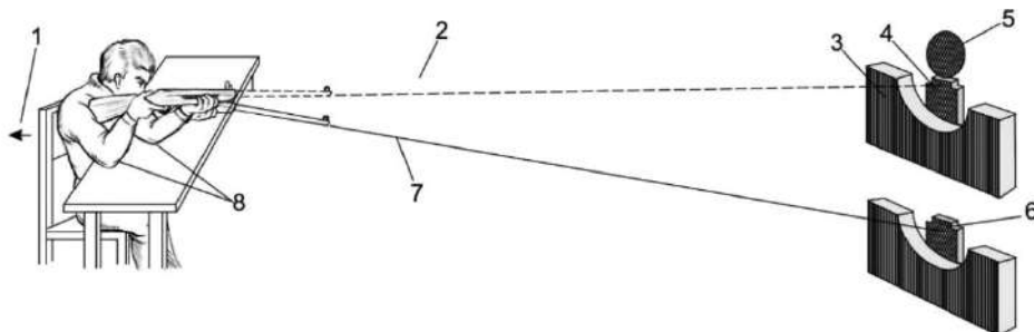
Іл. 21.4. Уточнення наведення гвинтівки по вертикалі під час стрільби сидячи за столом: 1 — напрямок переміщення корпусу стрільця; 2 — лінія прицілювання після уточнення наведення гвинтівки; 3 — розташування прицілу після уточнення наведення гвинтівки; 4 — суміщені точки наведення і прицілювання; 5 — «яблучко» мішені — виявилось вище; 6 — точка наведення гвинтівки до уточнення; 7 — лінія прицілювання до уточнення наведення гвинтівки; 8 — лікті стрільця мають бути нерухомі
